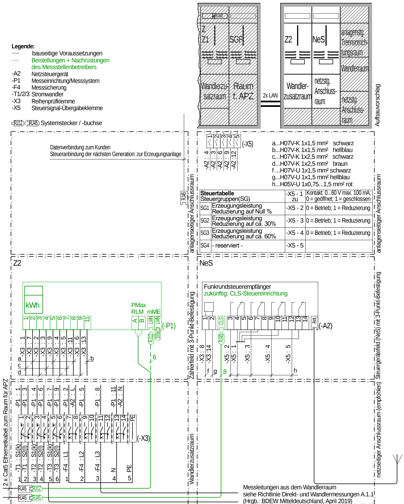
Bild 2 Aufbau Zählerplatz / NeS-Platz (Wandlermessung)
