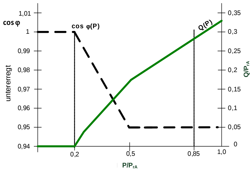
Bild 3 Q = f(P/P_{rA}) -Kennlinie für EZA mit P_{rA} \geq 135 \text{ kW} und Anschluss in den Umspannungsbereichen Königsbrück, Kamenz, Zescha, Kleinsaubernitz, Niesky, Görlitz und Weinhübel
